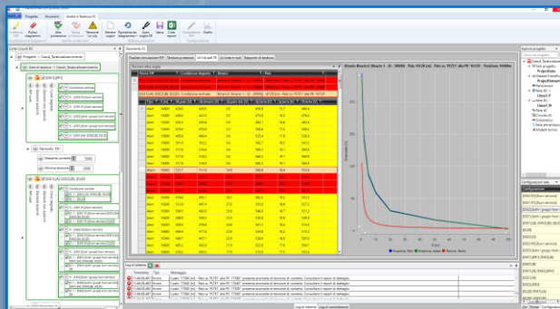
Verifica tensioni di passo e contatto
